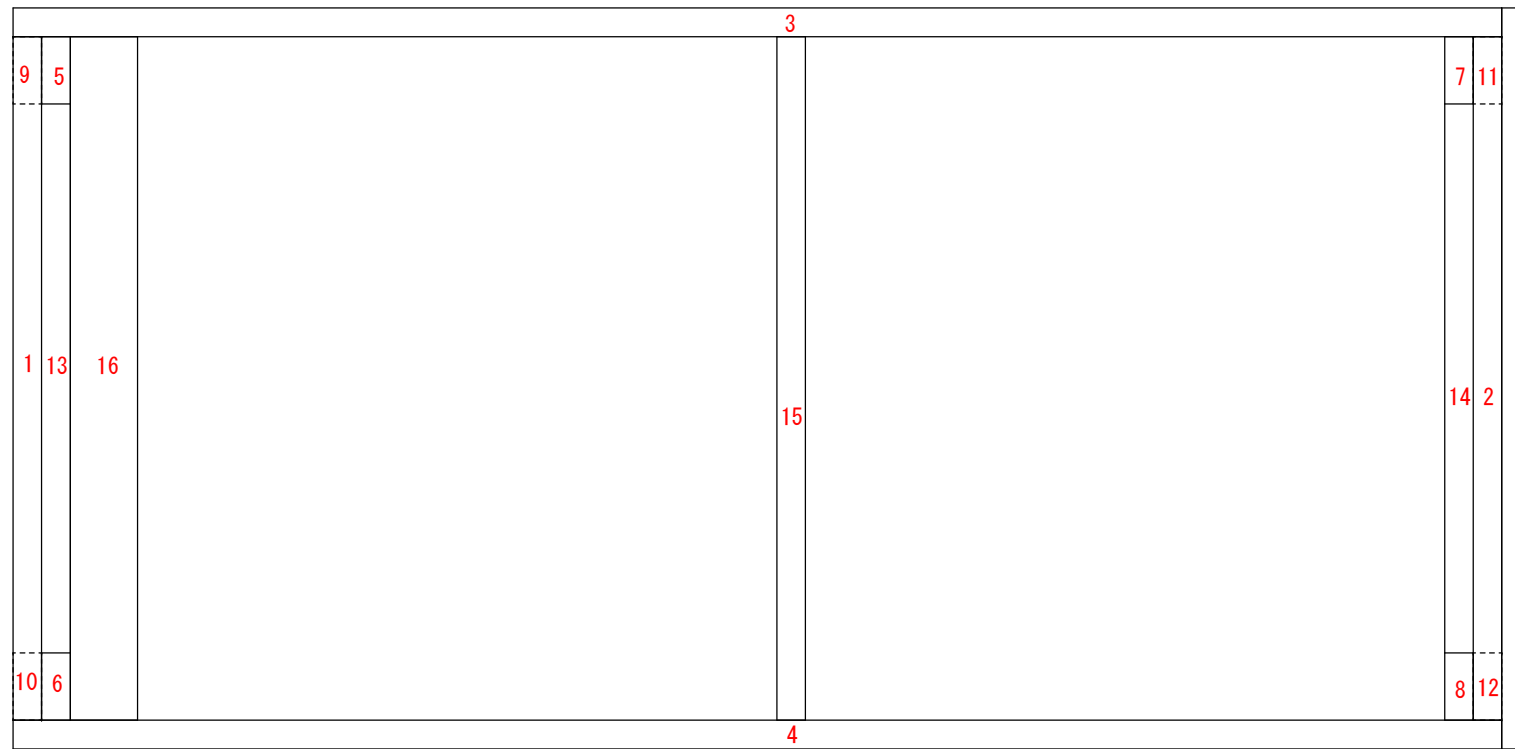
フレーム (全て2×4材)
